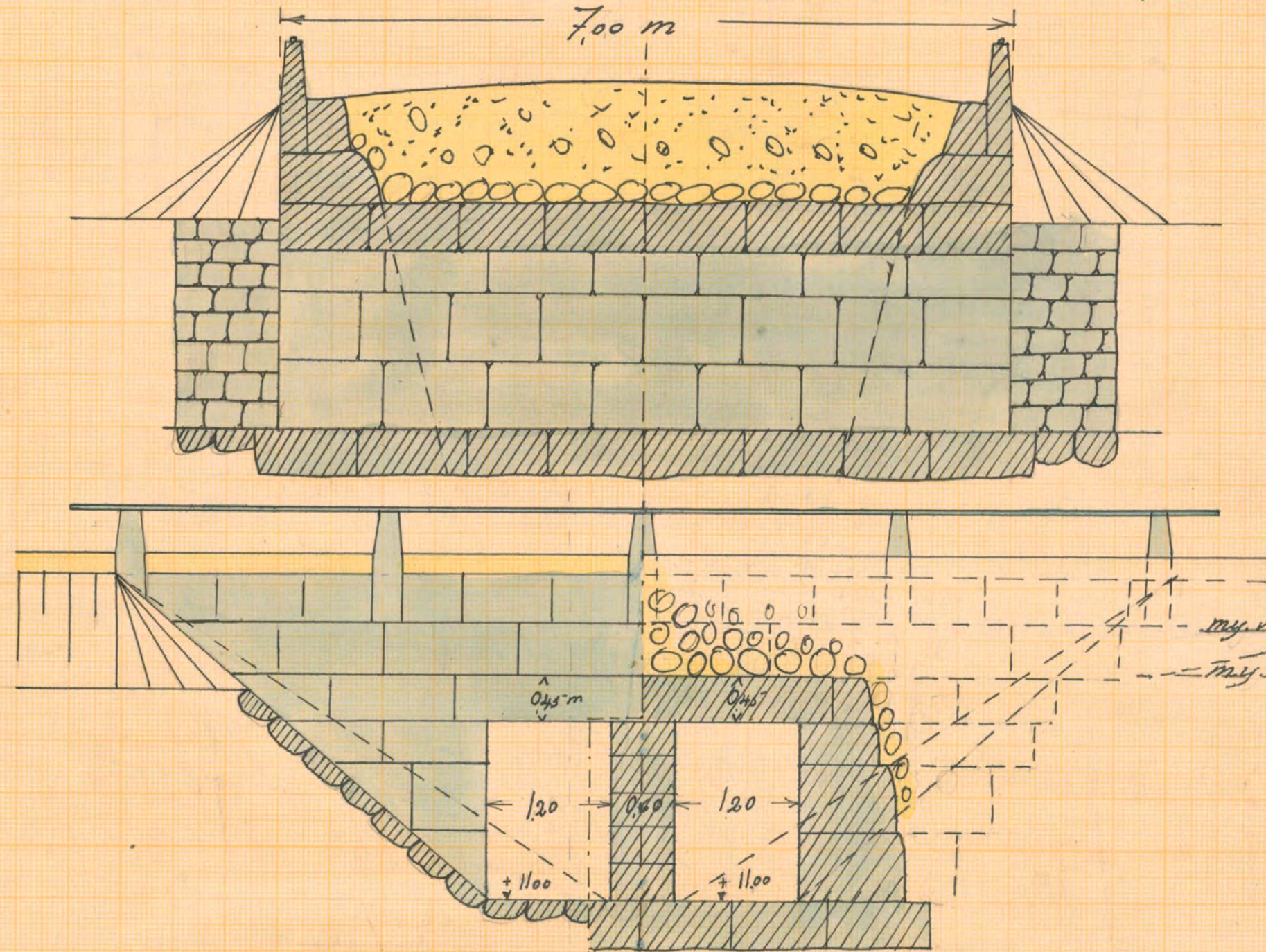
Förslag till Landsvägsbro vid 17+75
