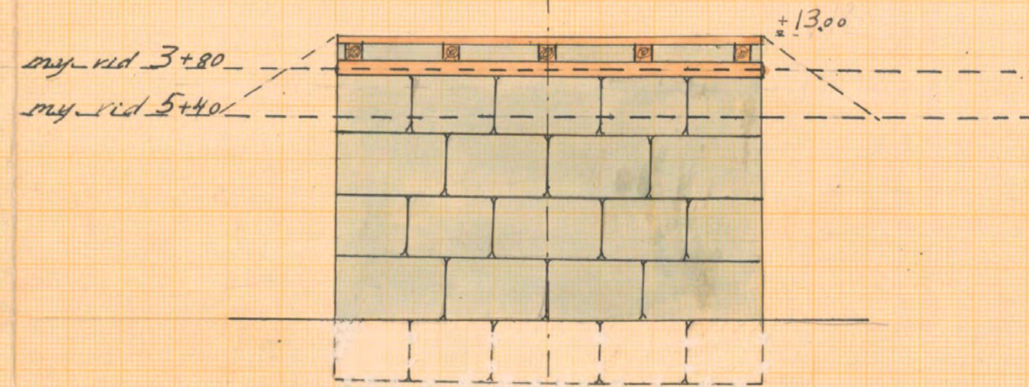
Förslag till ägrovägsbro vid 3+80 och 5+40
