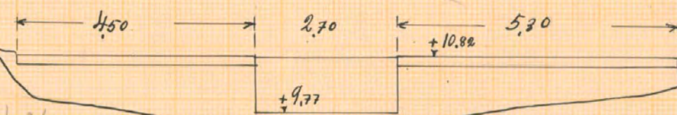
Landsräs bron vid 124,80
