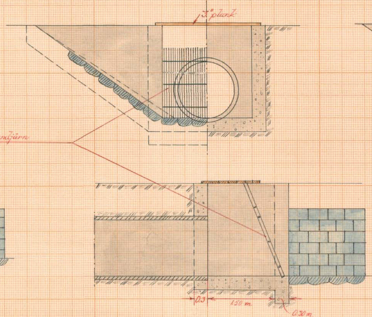
Intagningsbassäng vid p. 2 +00
