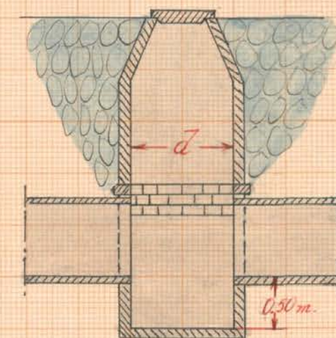
Intagningsbrunnar.
