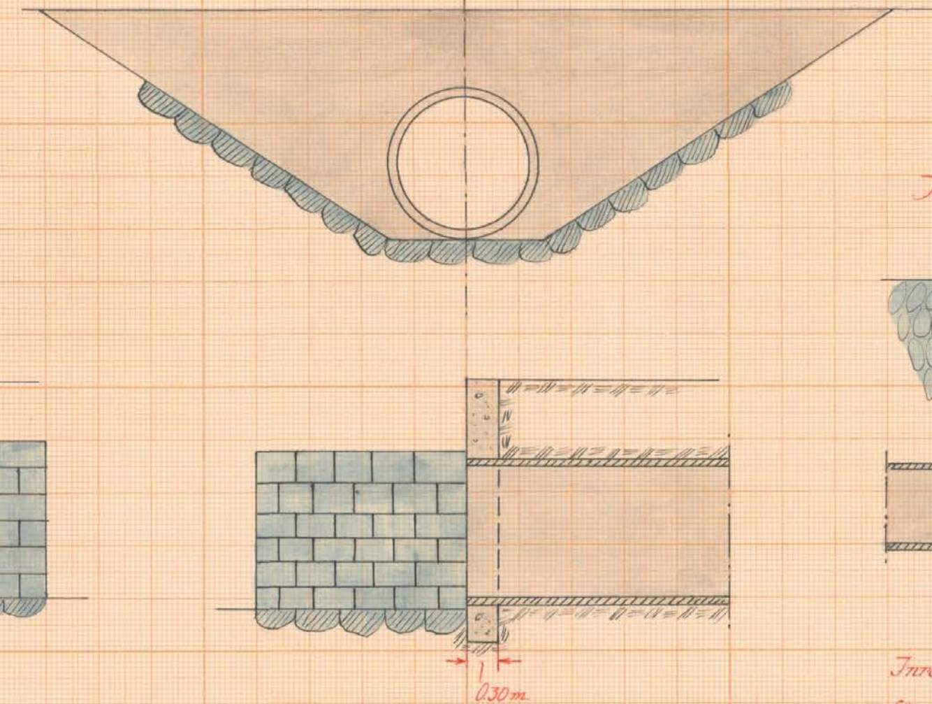
Dikesöga vid p. 6a +35 och 55 +00
