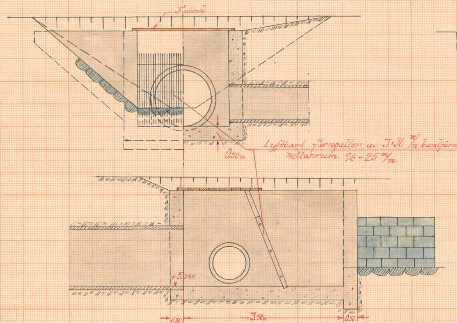
Intagningsbassäng vid p. 8 +62
