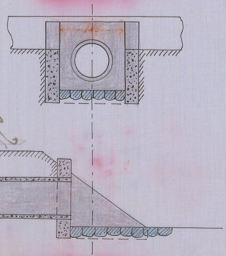
Förslag till dikeögon vid punkt C. Alternativ II.
