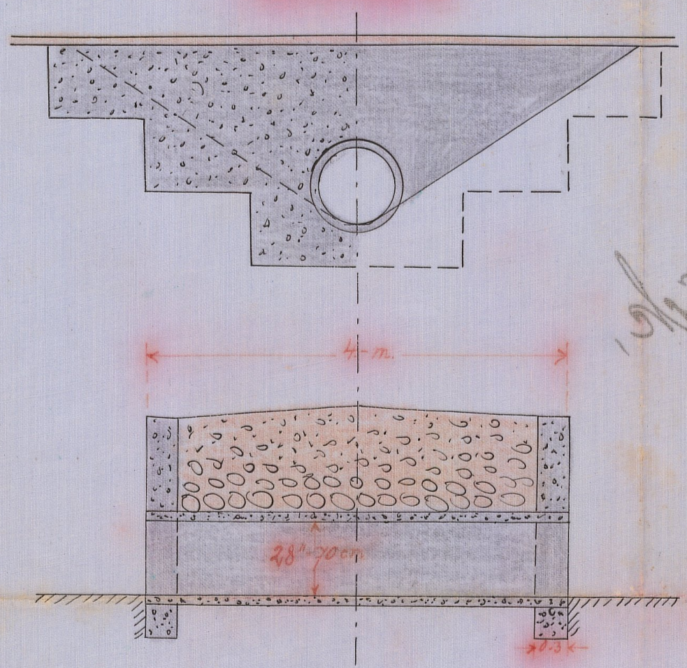
Förslag till ägrovägsbrunnar vid punkt 1+30 & 2+85. Alternativ I.
