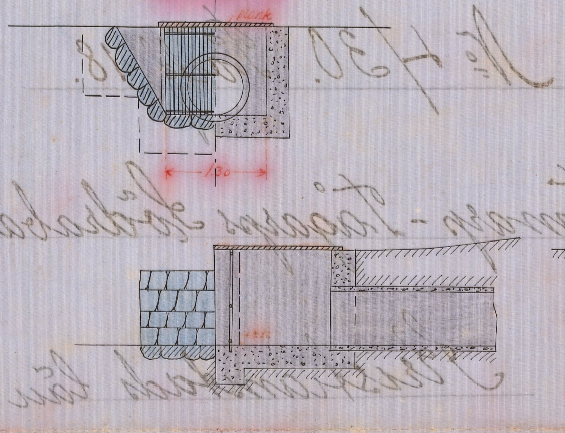
Förslag till intagningsbassäng vid punkt 7a+30 & 4+85. Alternativ II.
