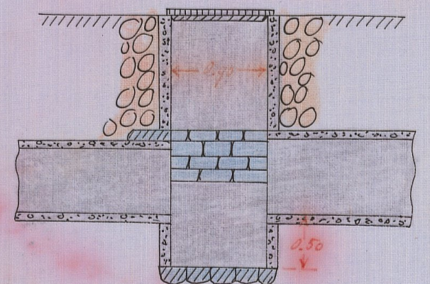
Förslag till intagningsbrunnar
