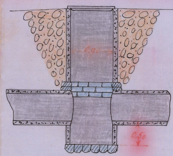
Förslag till inagångsbrunnar.
