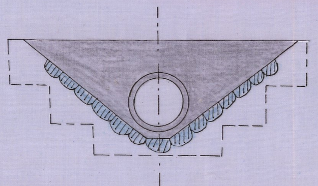
Förslag till åkesöga vid mark 0.
