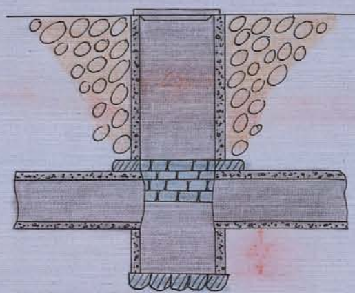
Förelag till intagningsbrunnar.
