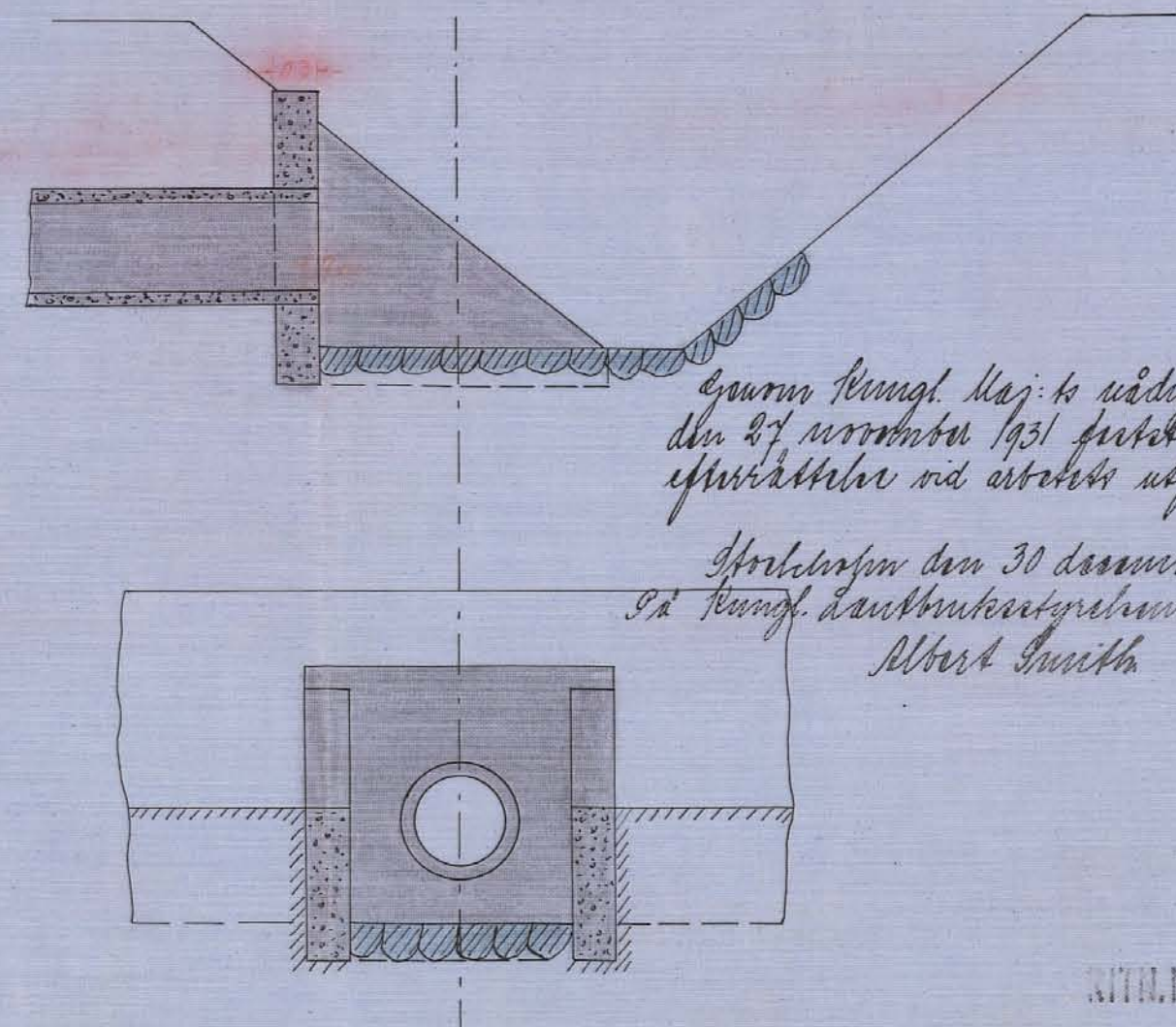
Förelag till dikesöga vid punkt C.
