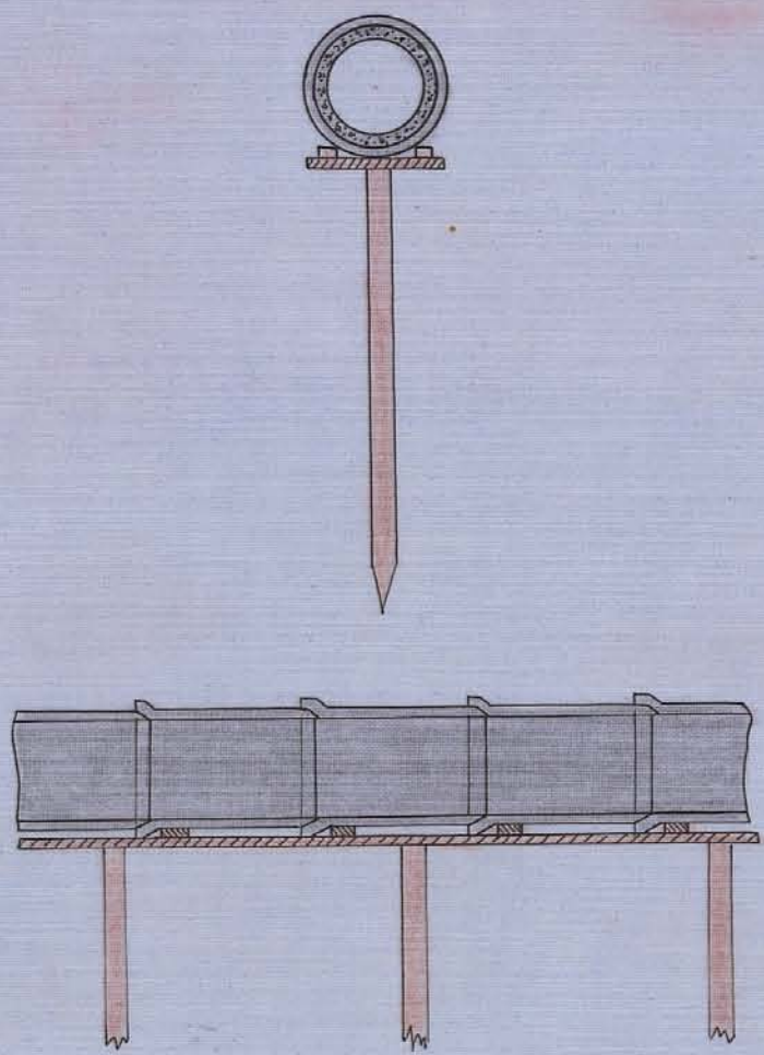
Förelag till rörens läggning på brädfotlar.
