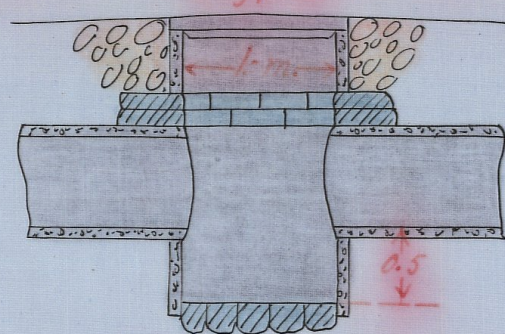
Förslag till ägervägskulvert vid punkt 0 30 Alt II.
