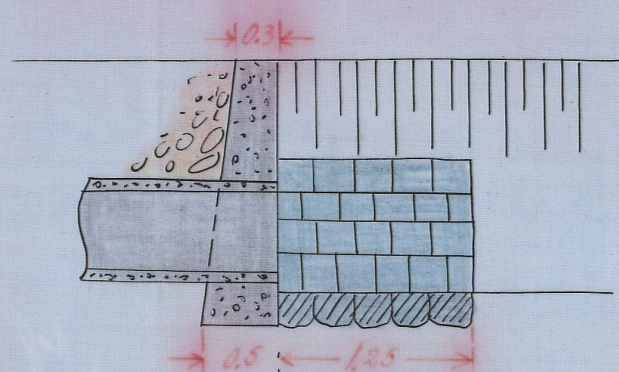
Förslag till dikesöga
