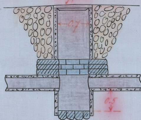
Förslag till dikesöga
