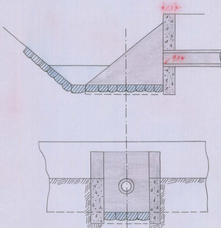
Förslag till dikesöga.
