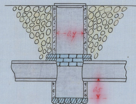
Förslag till intagningsbrunn
