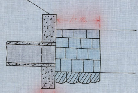
Förslag till intagingsbrunn
