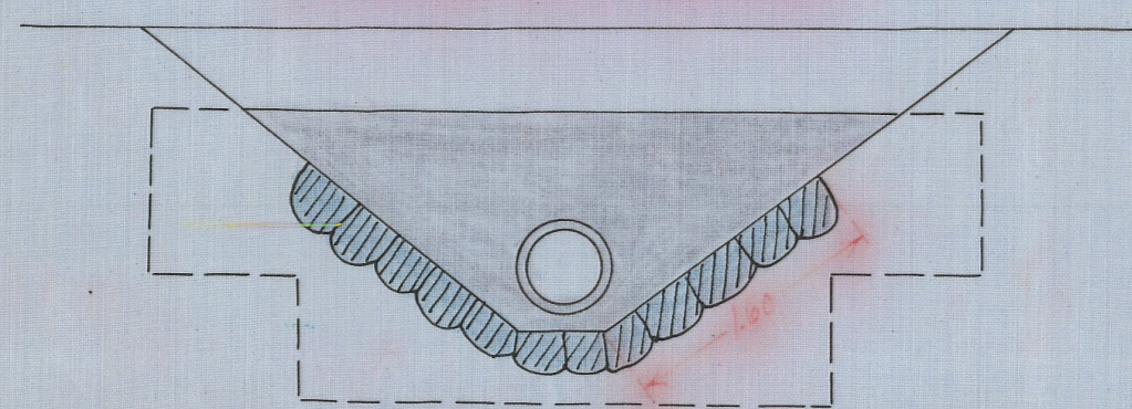
Förslag till dikesöga
