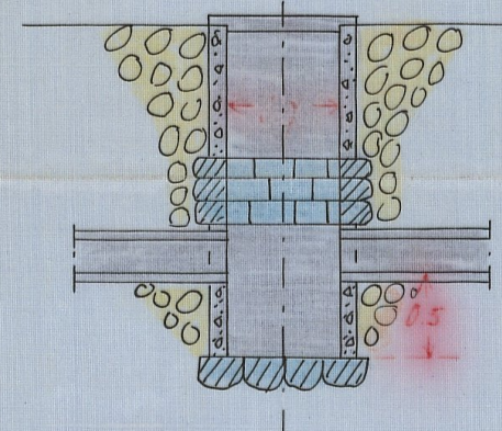
Förslag till intagningsbrunn.
