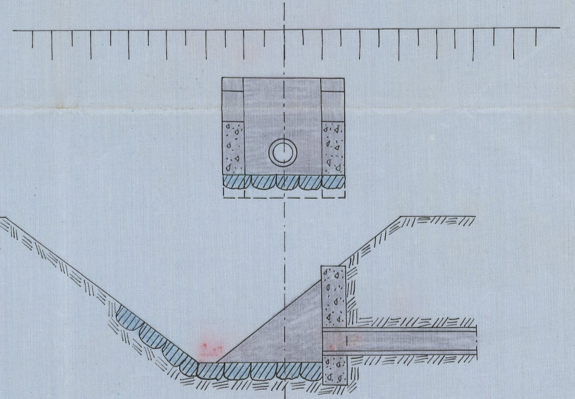
Förslag till dike-söga
