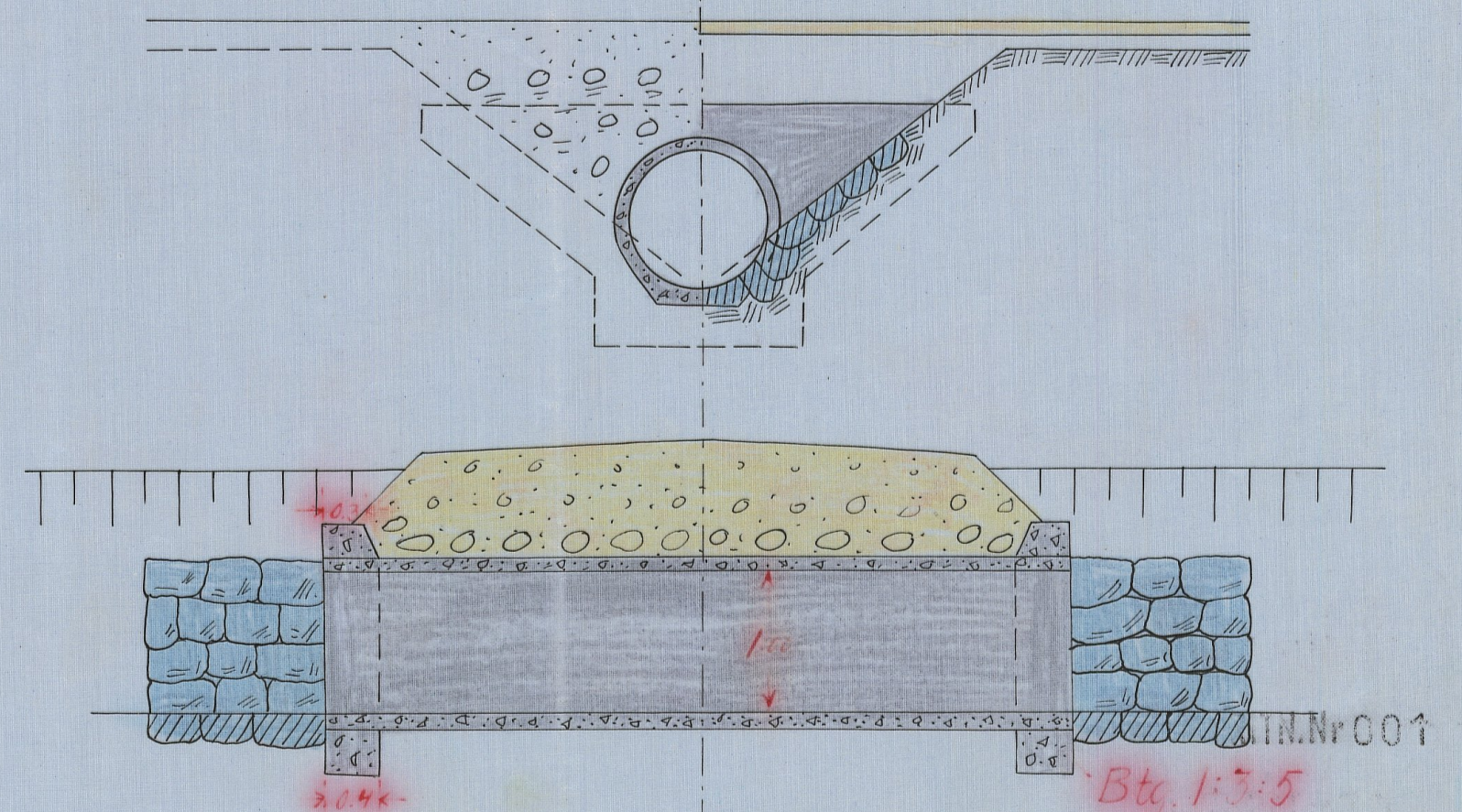
Förslag till ägovägstrumma
