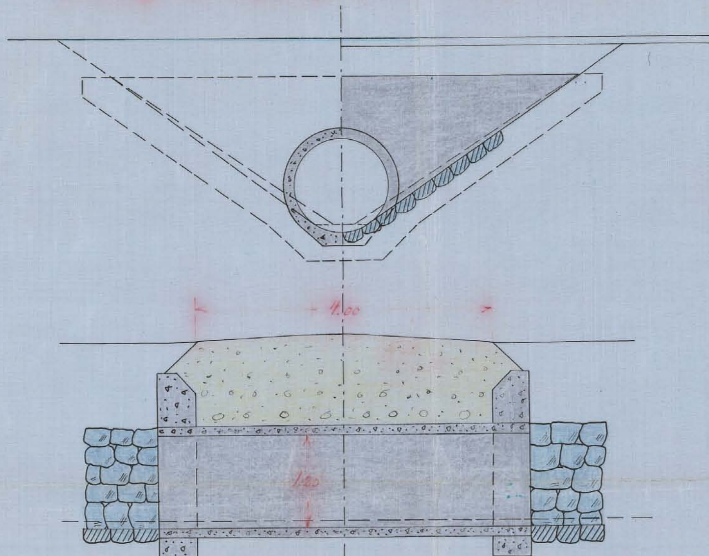
Förslag till ägrovägskulvert vid punkt 10 50
