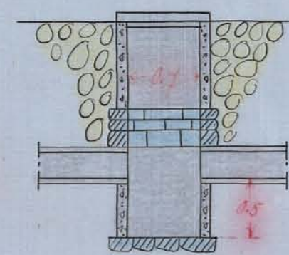
Förslag till intagningsrum
