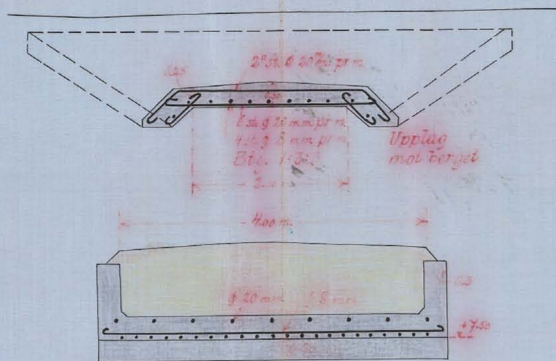
Förslag till ägrovägstro vid punkt 8 50
