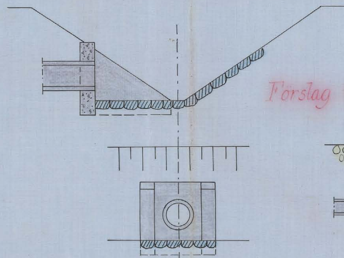
Förslag till dikesöga
