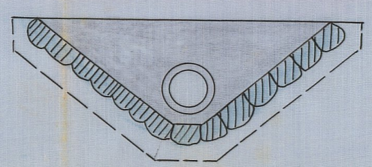
Förslag till dikeöga
