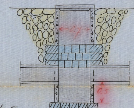
Förslag till vattenrörsbrunn
