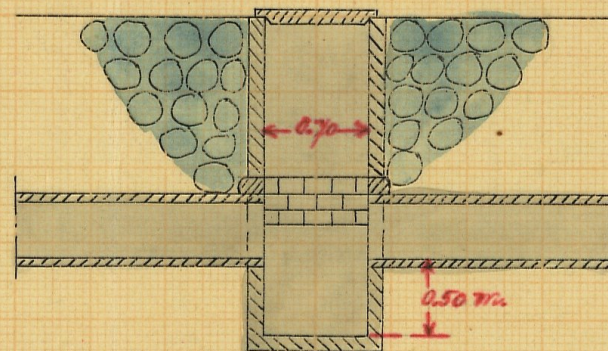
Intagningsbrunn vid 14+35
