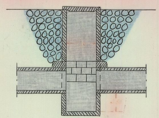
Förslag till vägringsbrunn
