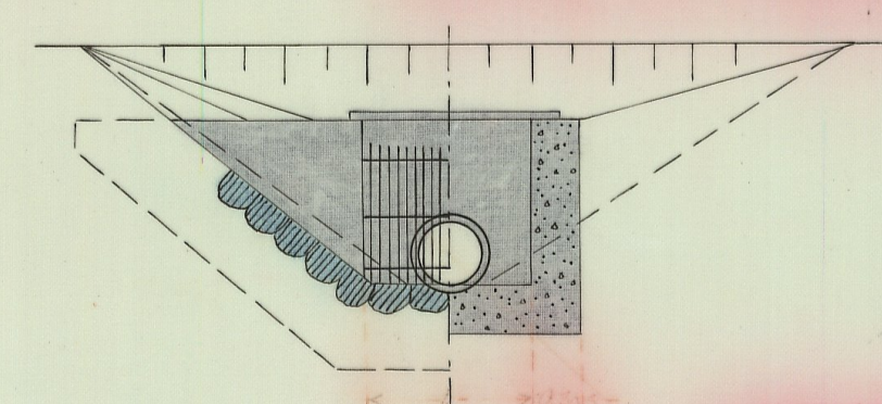
Förslag till vattningabassäng
