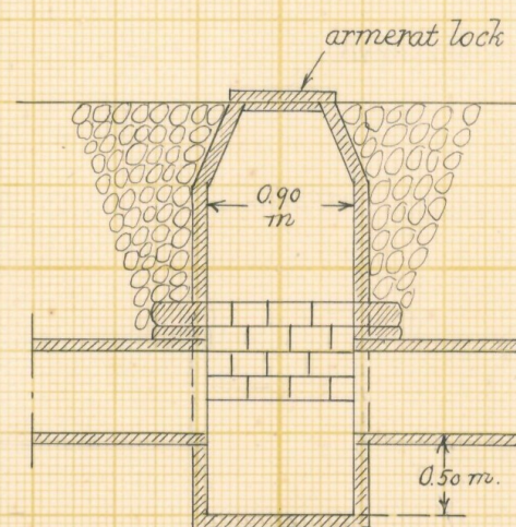
Typritning till intagningsbrunnar vid 20" rörledning vid 9" rörledning
