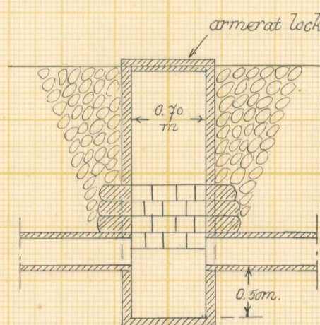
Typritning till intagningsbrunnar vid 20" rörledning vid 9" rörledning
