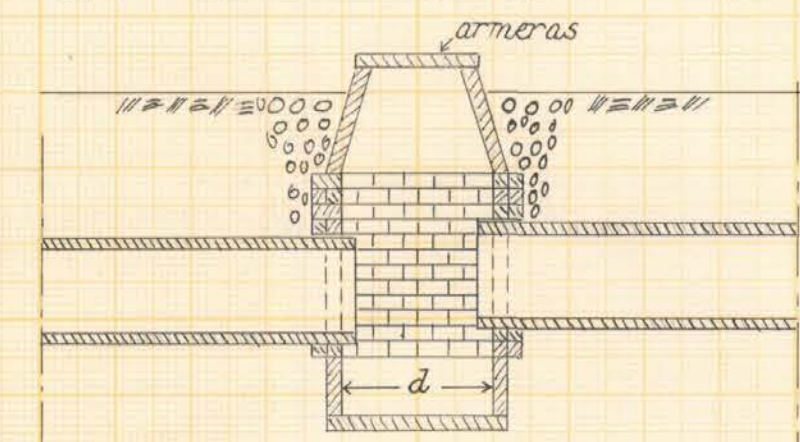
Typritning till intagningsbrunnar.
