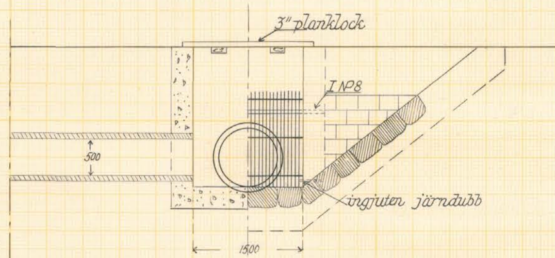
Förslag till intag vid C.
