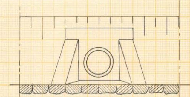
Förslag till utlopp vid D.
