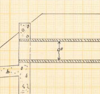
Förslag till utlopp vid D.
