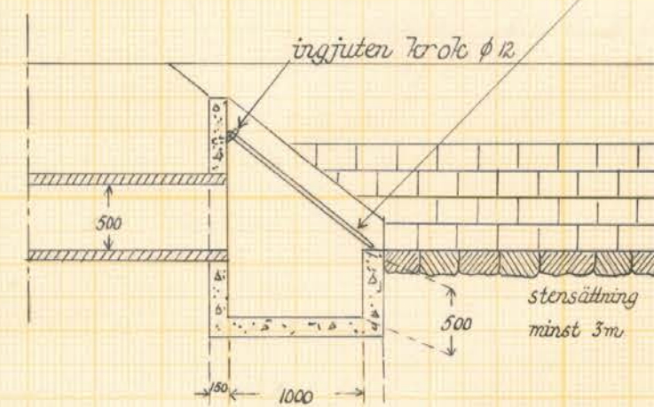
Ljftbart jängaller av plattjärn 4x40 mm % 50 mm
