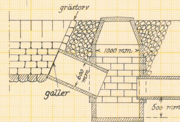
Förslag till intagningsbrunn vid 4 + 86.
