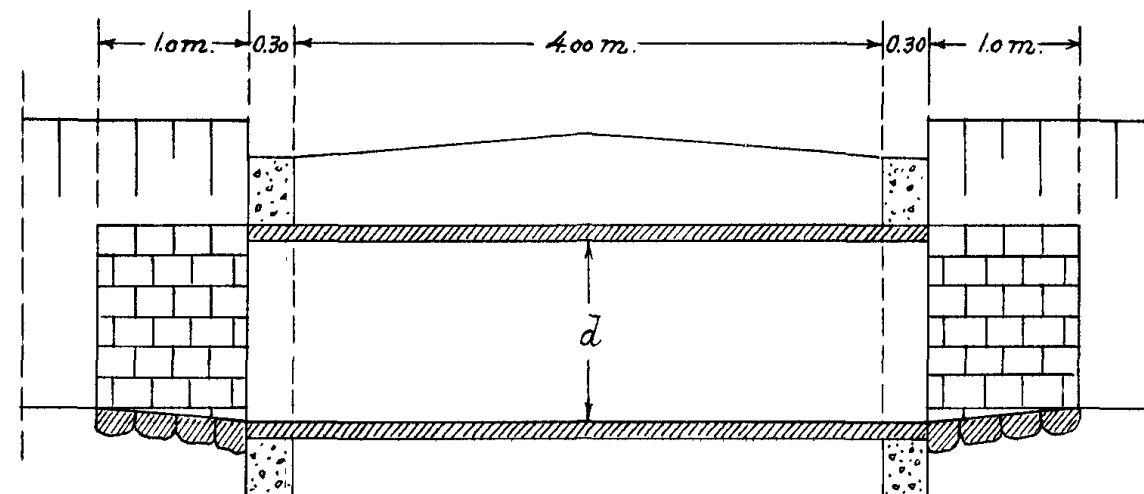
Typritning till rörtrummar vid 1+40, 7+15, 8+36 och 10+92.
