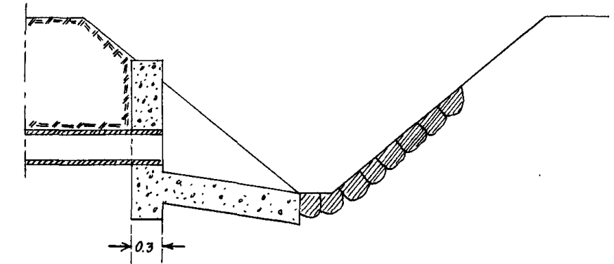
Typritning till utlopp vid 30 och 50.
