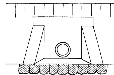
Typritning till utlopp vid 30 och 50.
