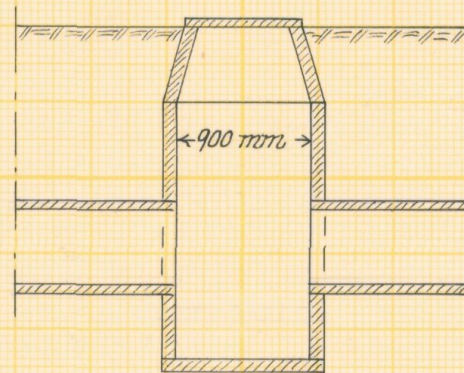
Typritning till brunnar i sträckan A-B-C-D.
