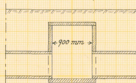
Förslag till brunn i punkt 8+00.
