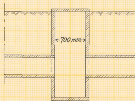
Förslag till brunn i punkt 20+64.
