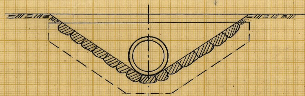
Typritning för rörutlopp vid 4+38 och 6+72
