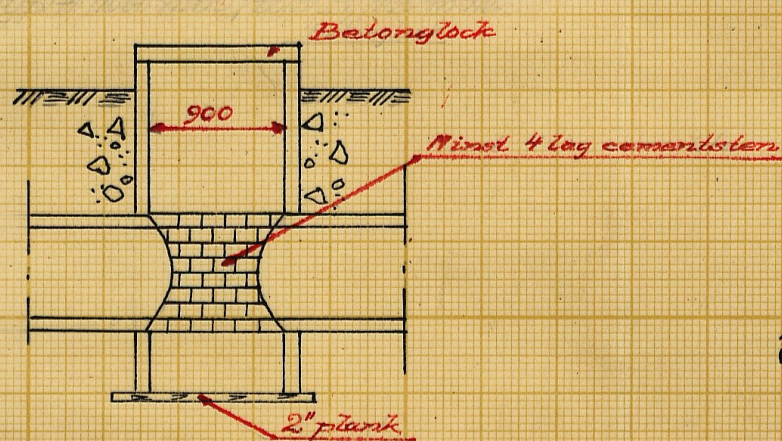
Typritning för brunnar Typ A 1000 mm, typ B 900 mm.
