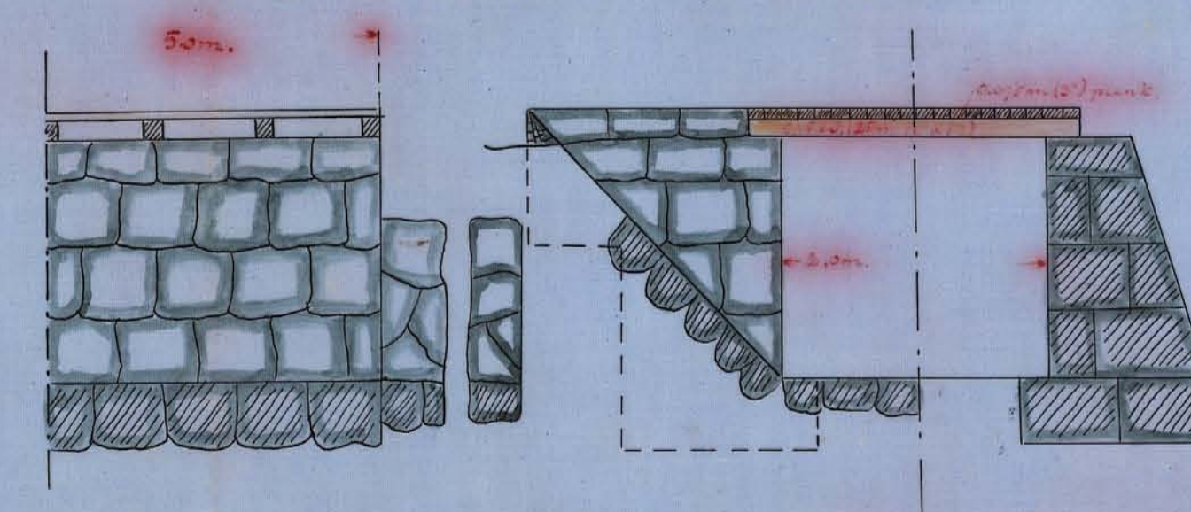
Förslag till ägövägsbro med stenlandfästen. Sk. 1:50
