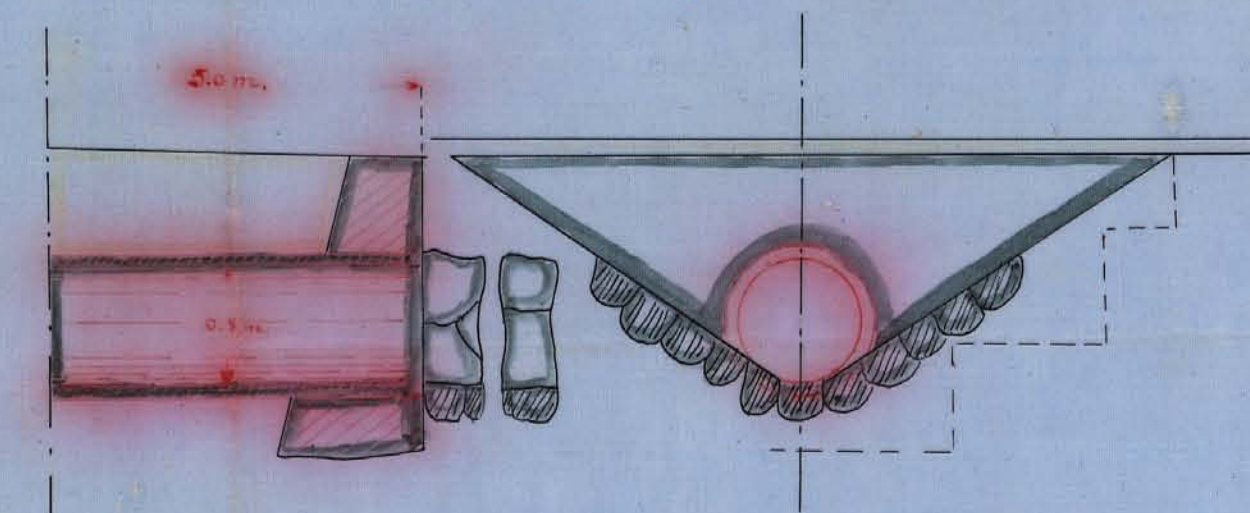
Förslag till ägövägsbro vid 60+40. Sk. 1:50
