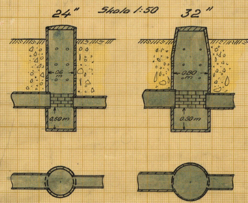
Typritningar för brunnar med inre diameter av:
