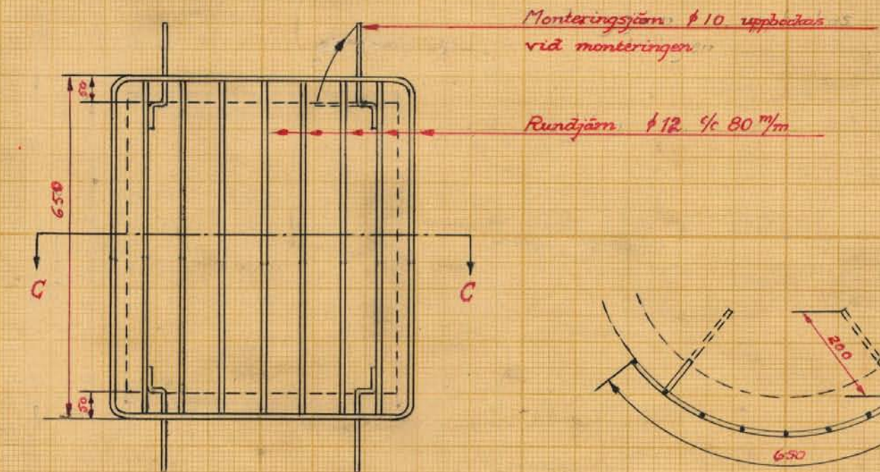
Detalj av galler skala 1:10
