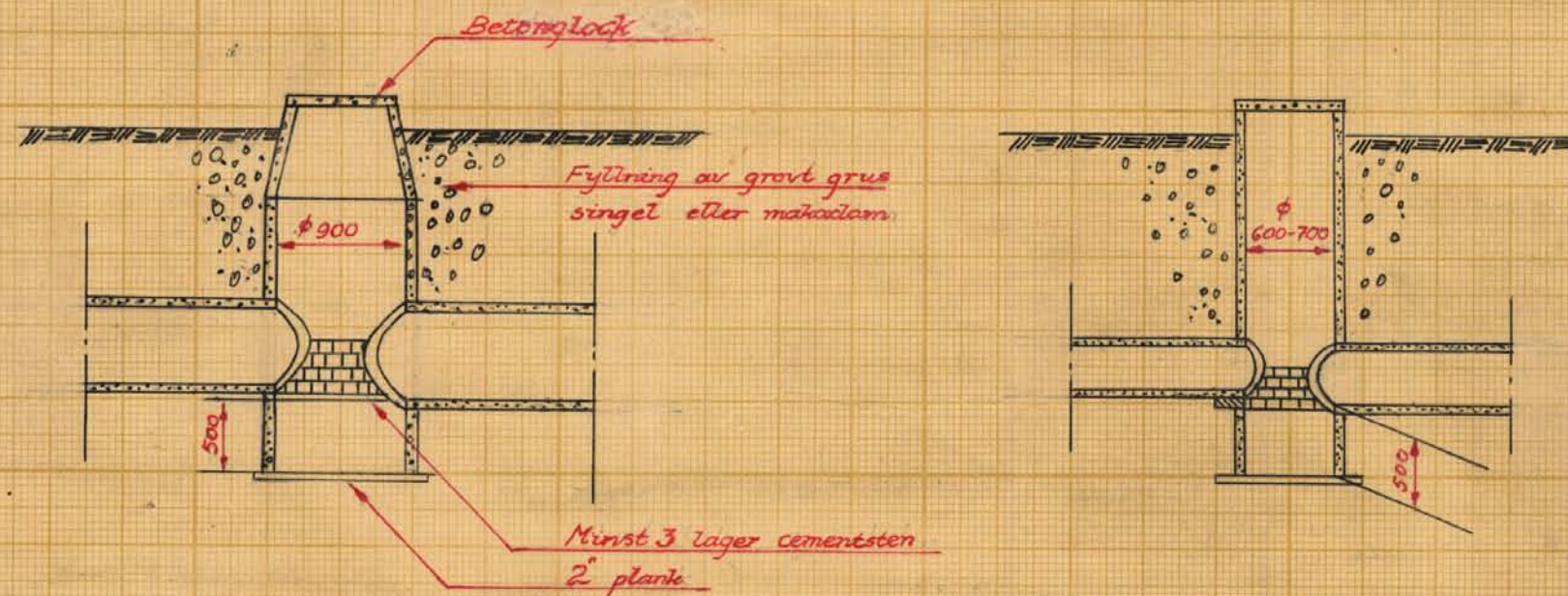
Typritning för brunnar
