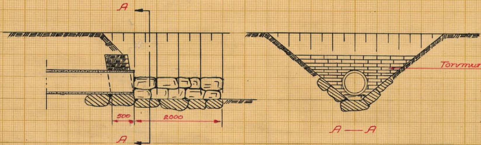
Typritning för rörutlopp
