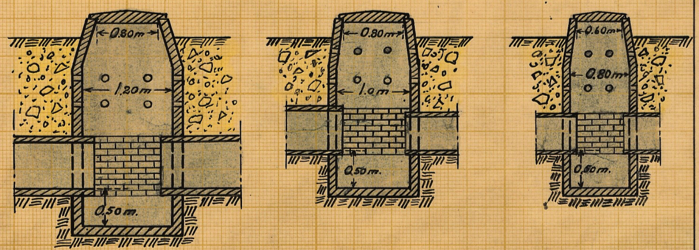
Typritningar för brunnar med inre diameter av: 48" 40" 32" Skala 1:50
