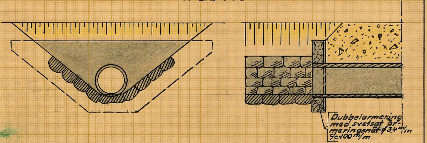
Typritningar för brunnar med inre diameter av: 48" 40" 32" Skala 1:50
