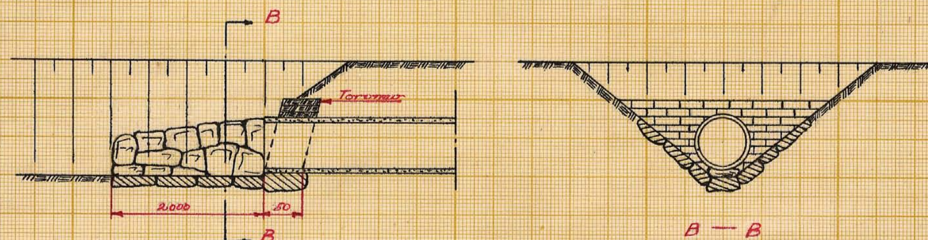
Typritning för rörutlopp
