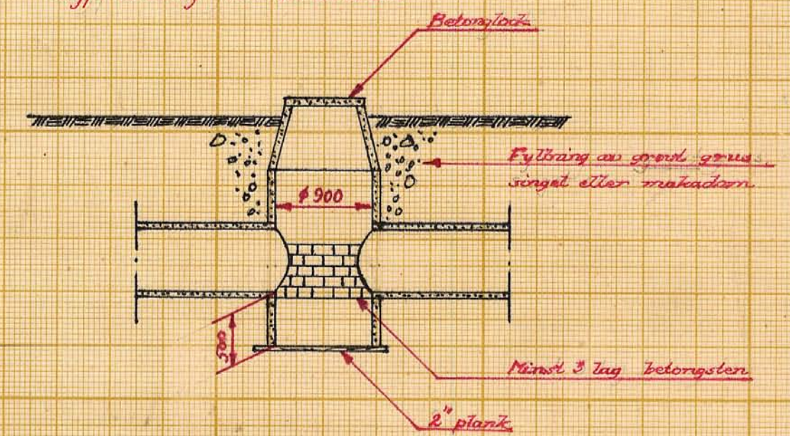
Typritning för brunnar
