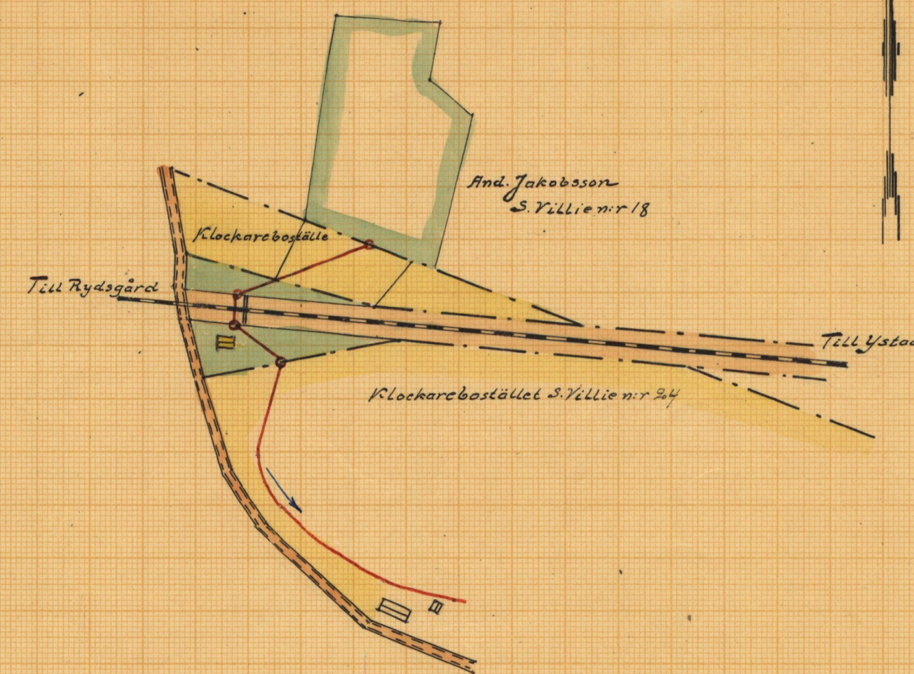
Situationsplan. Sk. 1:2000
