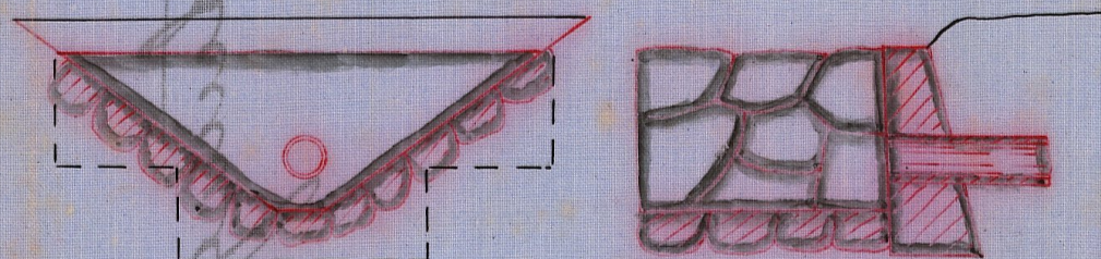
Förslag till ommurning av utlopp. Sk. 1:50.
