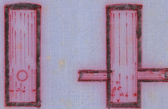
Förslag till ommurning av utlopp. Sk. 1:50.
