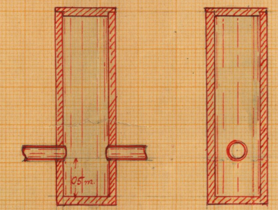
Förslag till brunn. Sk=1:50
