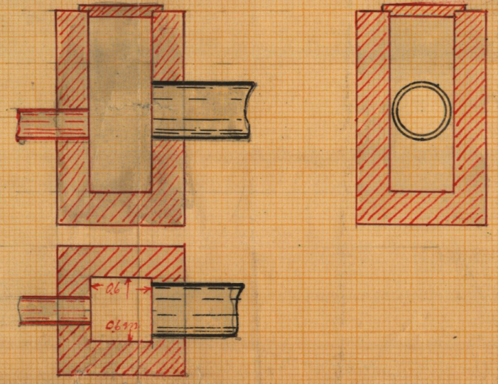
Förslag till brunn vid 3+40. Sk=1:50
