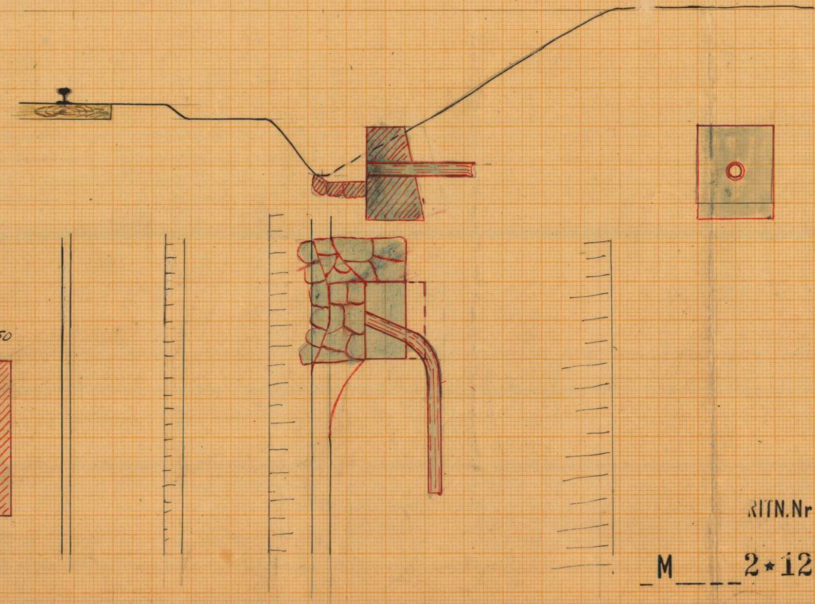
Förslag till kringmurning av utloppet vid F. Skala=1:50
