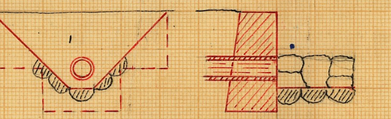
Förslag till kringmurning vid C skala 1:50
