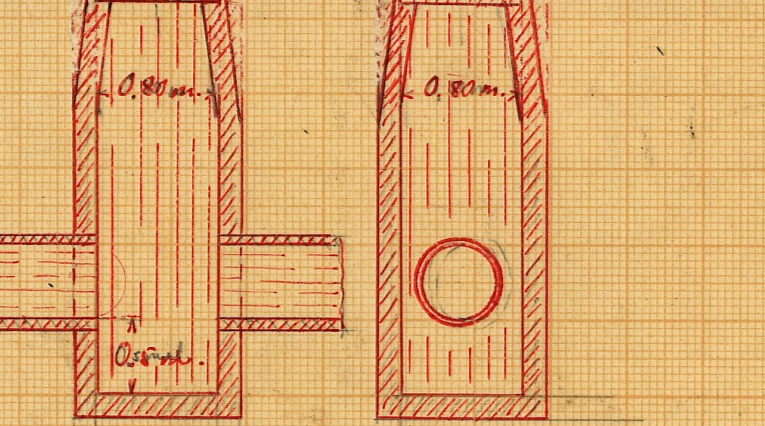
Förslag till brunn 10 m. d. d. m. skala 1:50
