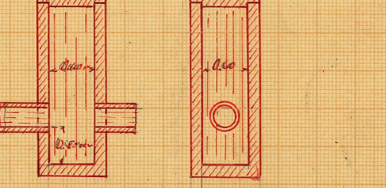
Förslag till brunn 10 m. d. d. m. skala 1:50
