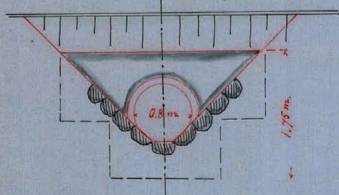
Förslag till ägövägsbro av 0.8 m. rör. Skala 1:50
