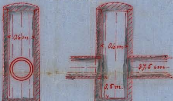
Förslag till brunn. Skala 1:50
