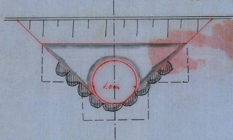
Förslag till ägövägsbro vid 5+68 Skala 1:50
