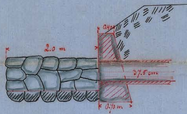
Förslag till kringmurning av utloppsörret vid 60 Skala 1:50
