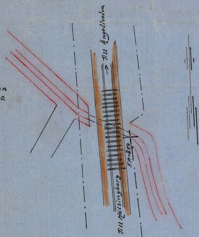
Förslag till ägövägsbro av 0.8 m. rör. Skala 1:50
