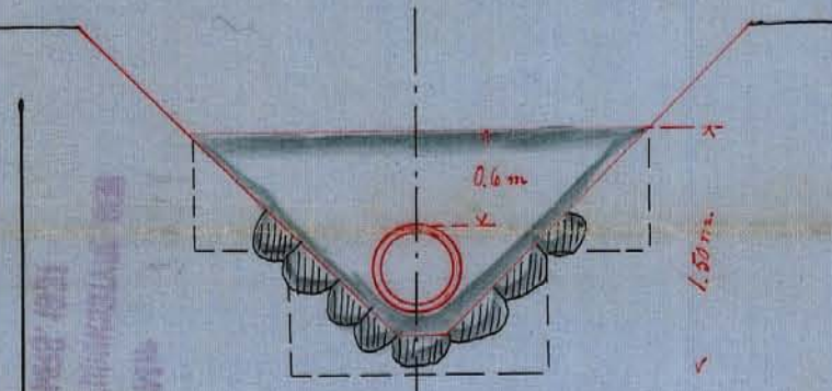
Förslag till kringmurning av utloppsörret vid 60 Skala 1:50
