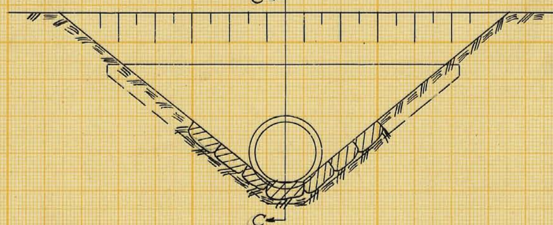
Sektion B-B
