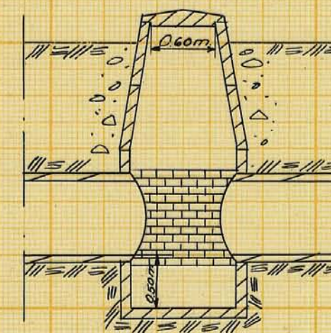
Förslag till 40" brunn Skala 1:50
