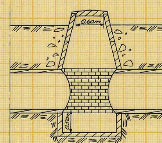
Förslag till 48" brunn Skala 1:50
