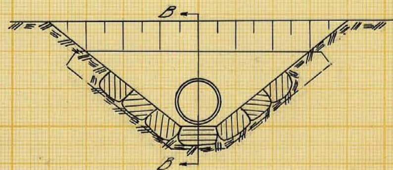
Förslag till ommurning av rörutlopp vid 0+16 Skala 1:50 Sektion A-A
