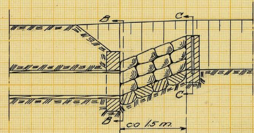
Förslag till ommurning av rörintag med galler vid 7 Skala 1:50 Sektion A-A
