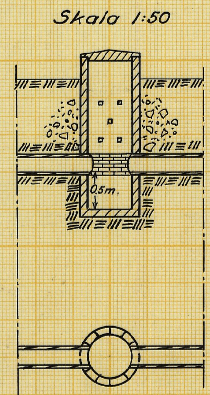
Förslag till 24" brunn.
