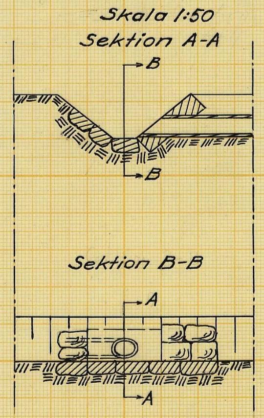
Förslag till ommurning av rörutlopp vid 3+92
