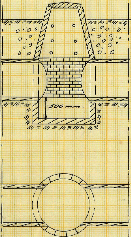
Typritning för brunn \phi 1200 . Skala 1:50.
