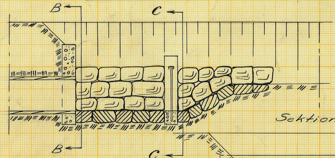
Sektion A-A.
