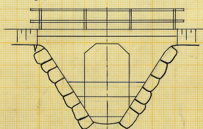
Bro för väg 1319 mellan 84+47=6+32-6+40.
