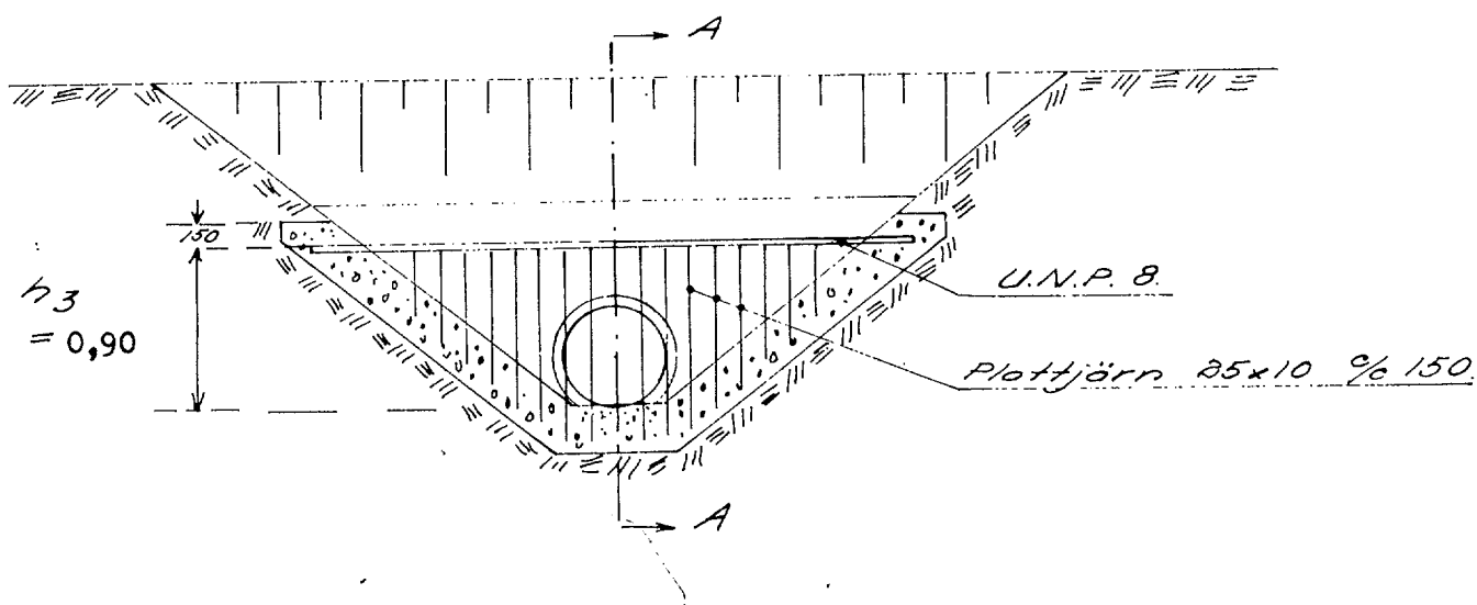
Sektion C-C.
