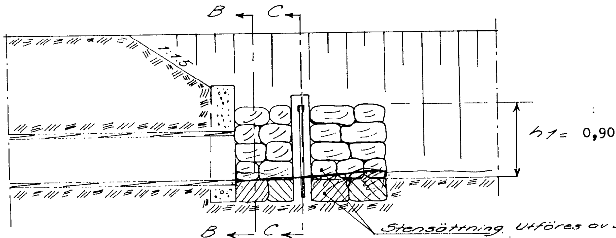
Sektion A-A.
