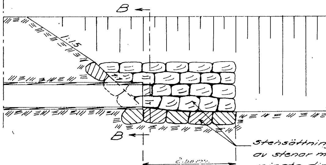
Sektion A-A.
