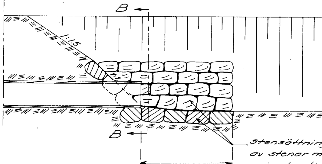
Sektion A-A.
