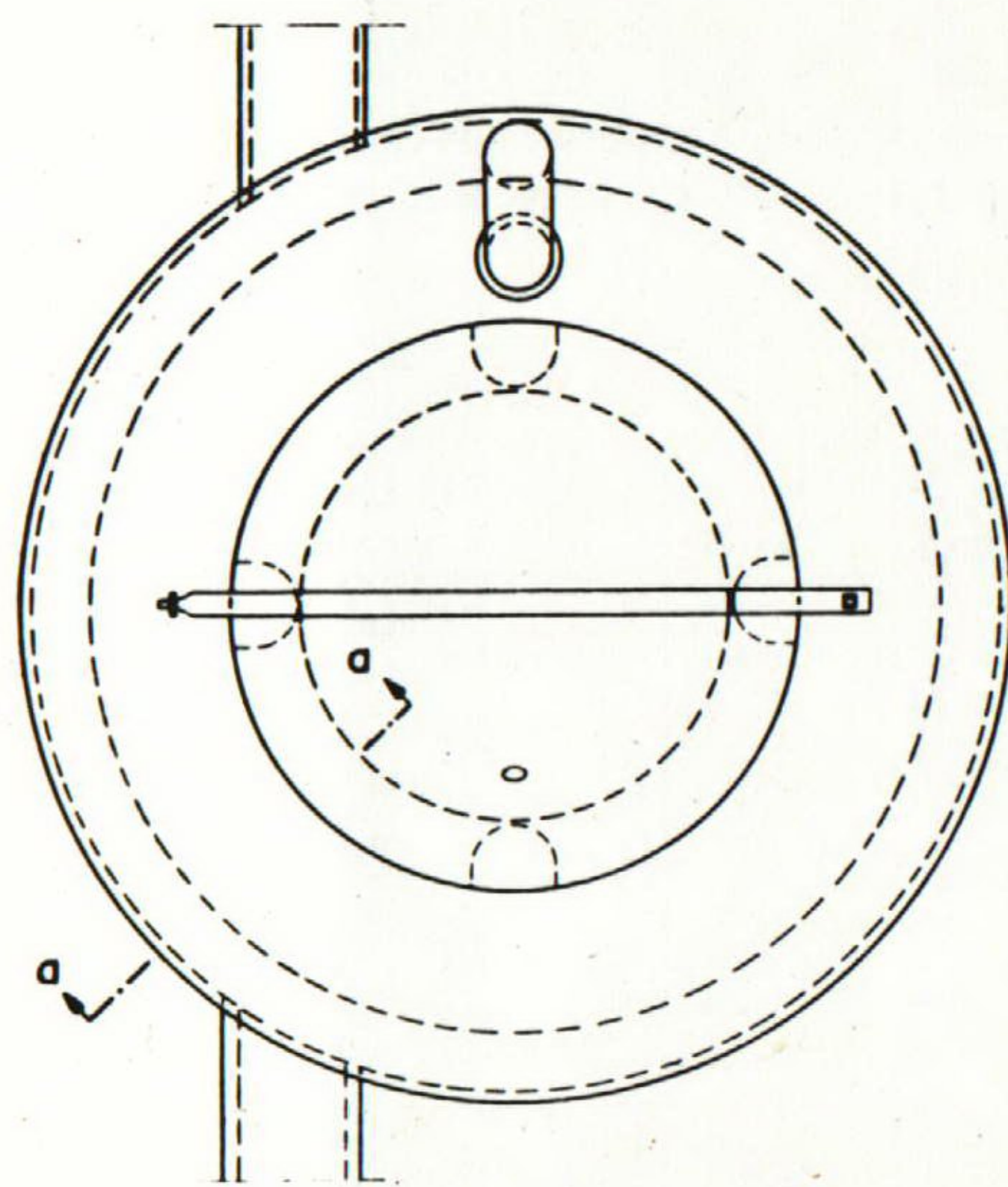
Sektion a-a
