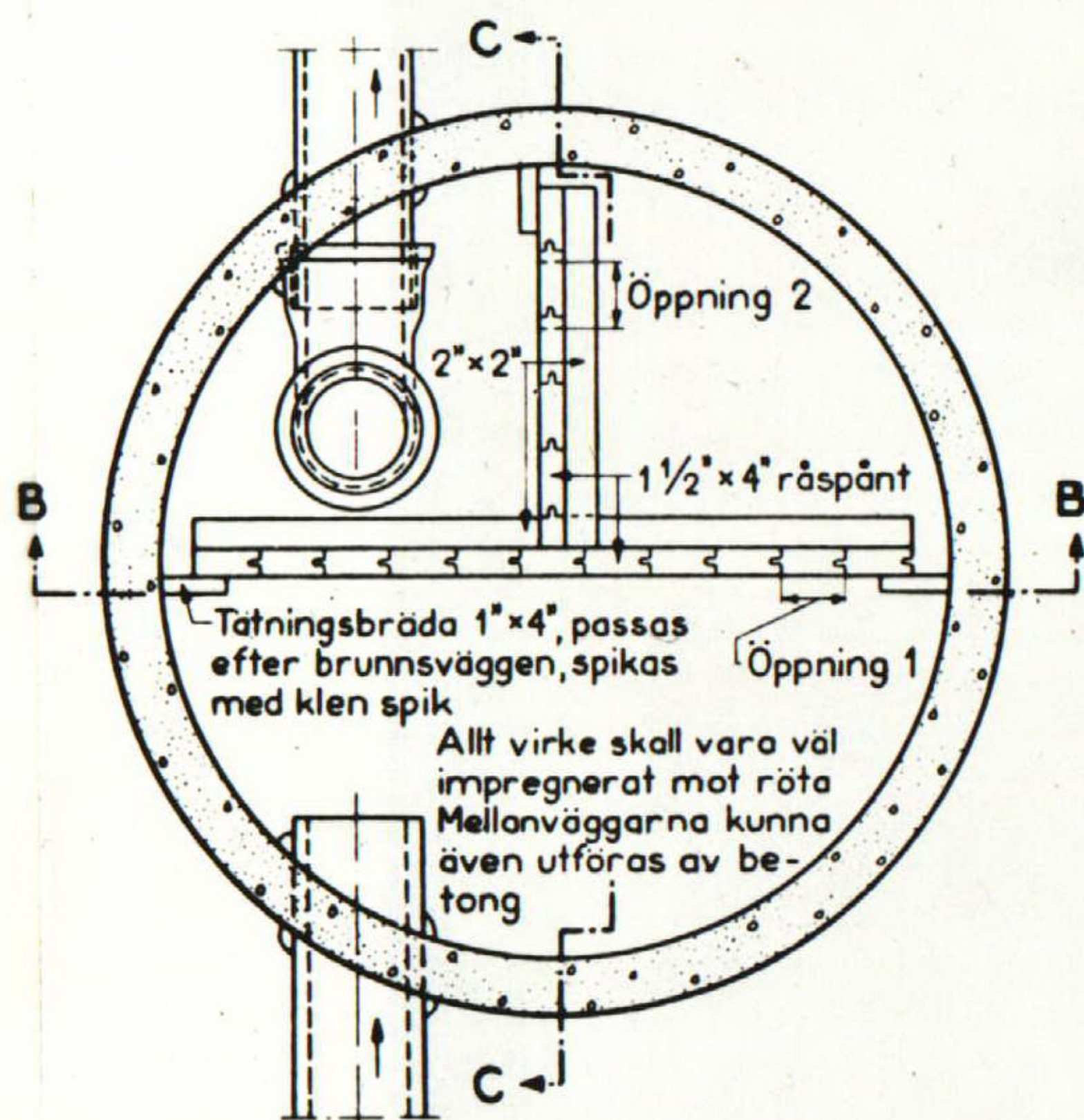
Plansektion A-A
