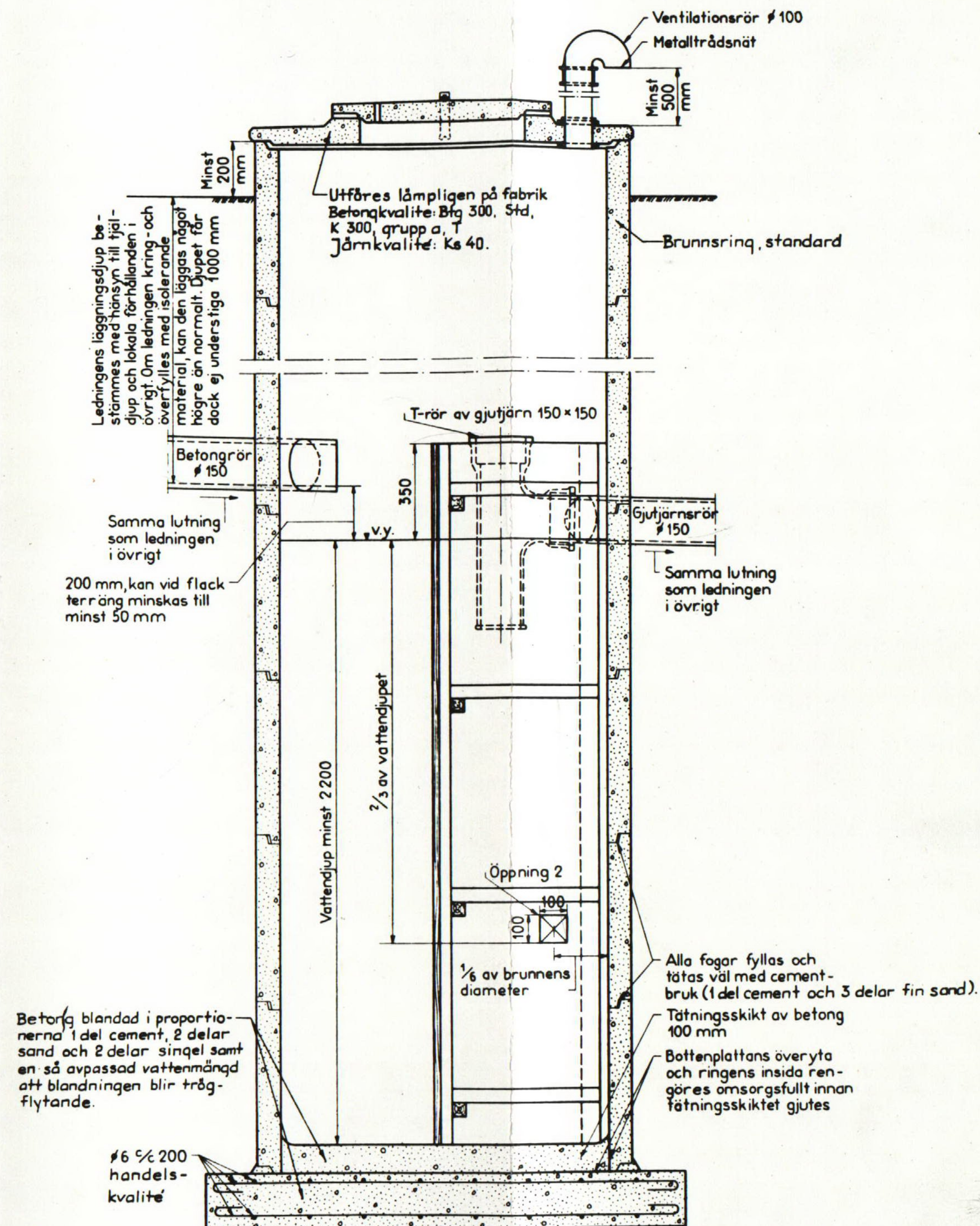
Slamavskiljare för avlopp från bebyggelse med upp till 10 invånare
