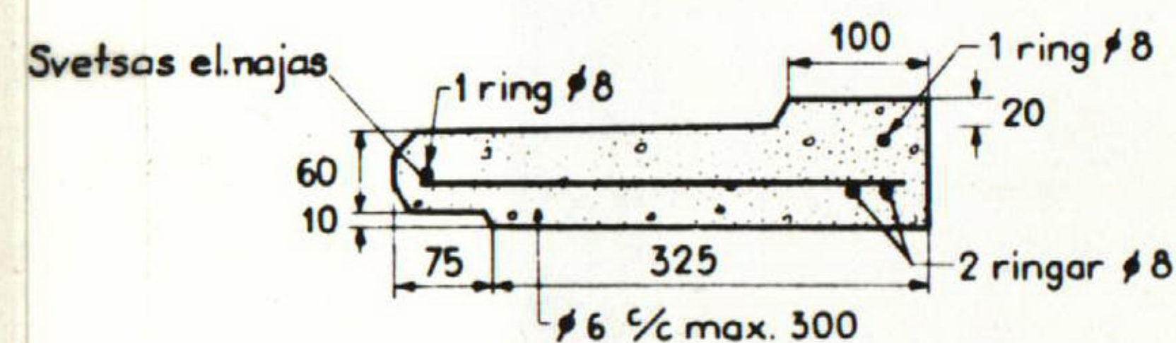
Plansektion A-A
