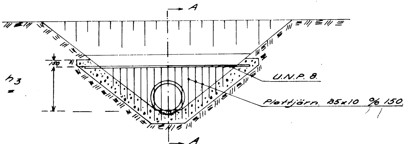
Sektion C-C.
