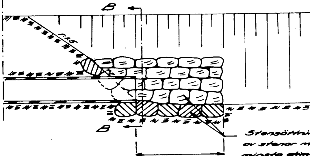
Sektion A-A.
