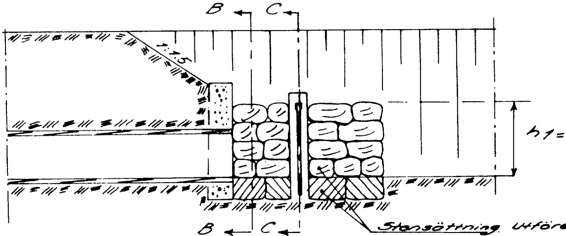
Sektion A-A.
