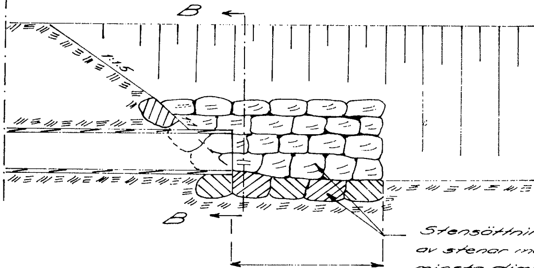
Sektion A-A.
