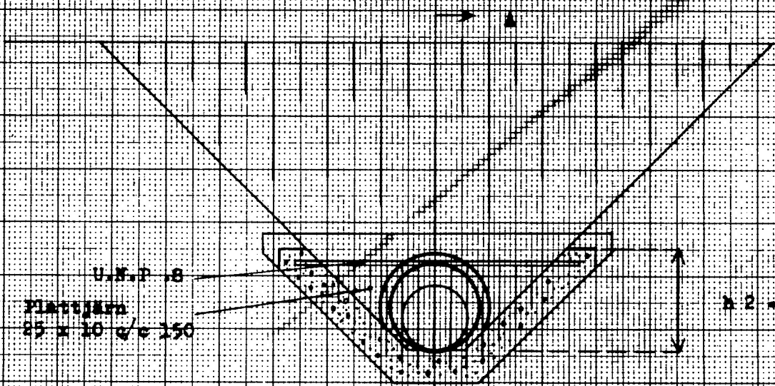
Sektion C - C
