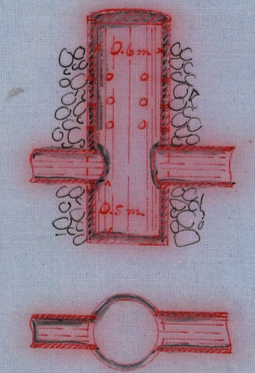
Förslag till brunn. Sk. = 1:50.
