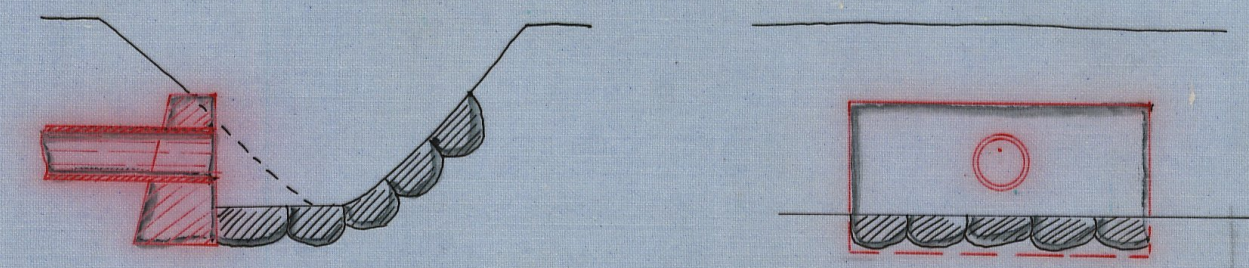
Förslag till ommurning av utlopp. Sk. = 1:50.
