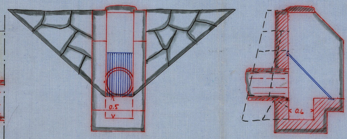
Förslag till indrag. Skala 1:50.
