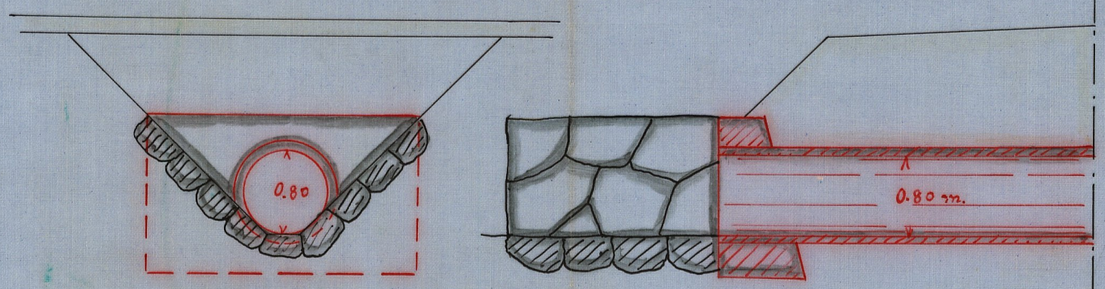
Förslag till brunn. Skala 1:50.
