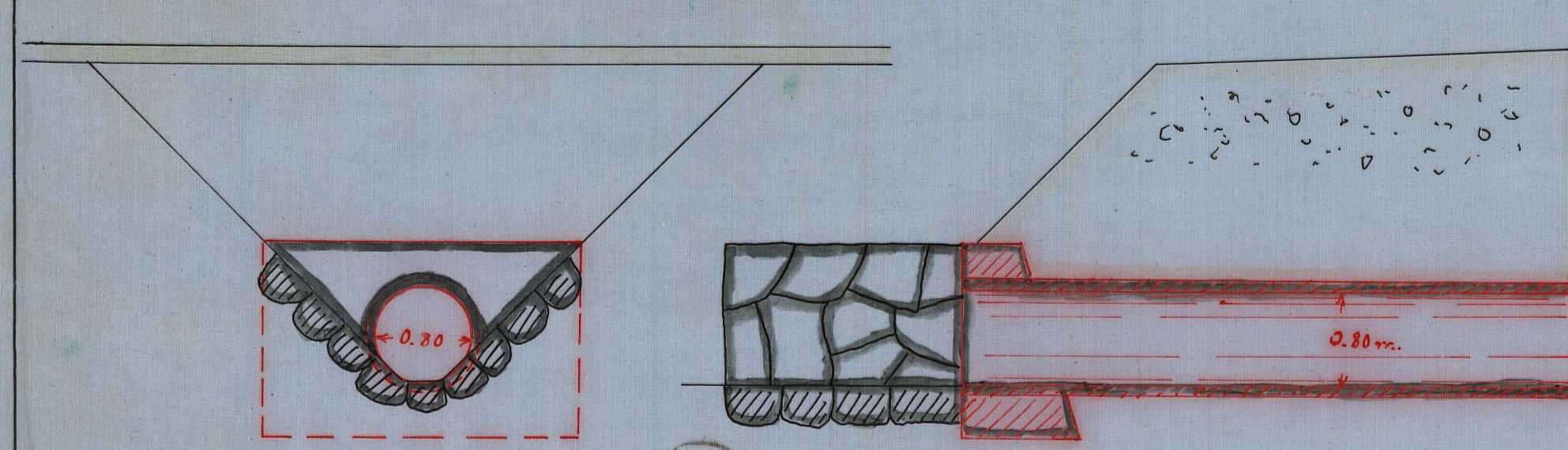
Förslag till brumma vid 4+23. Skala 1:50.
