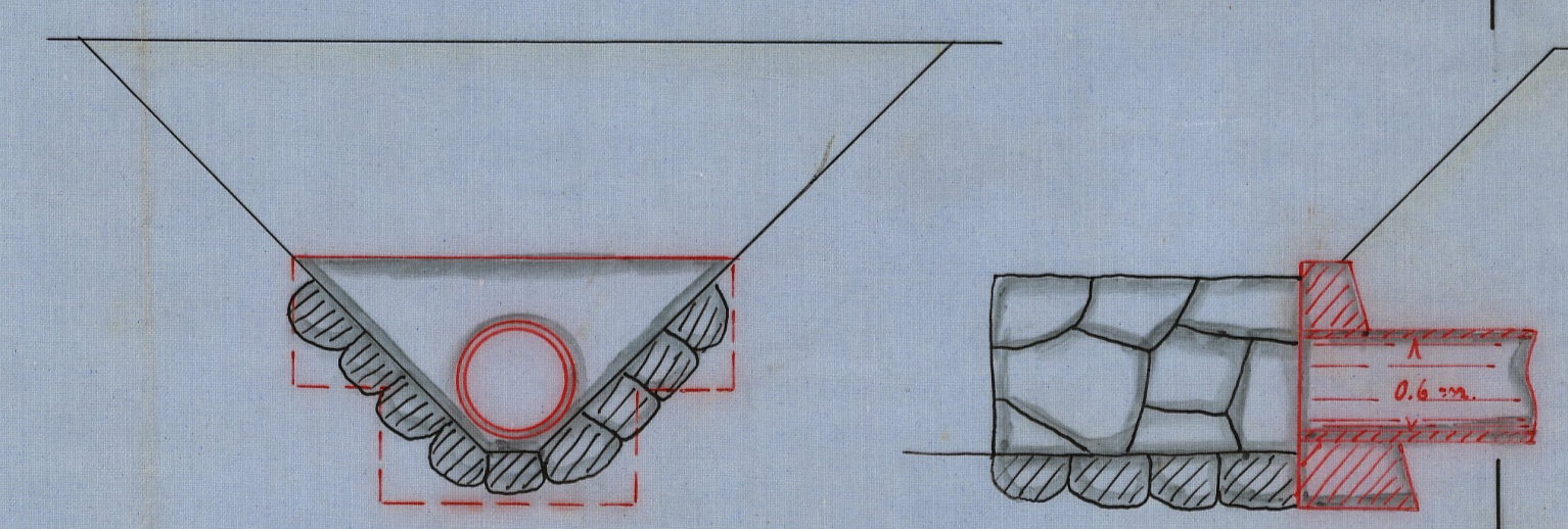
Förslag till omringning. Skala 1:50.
