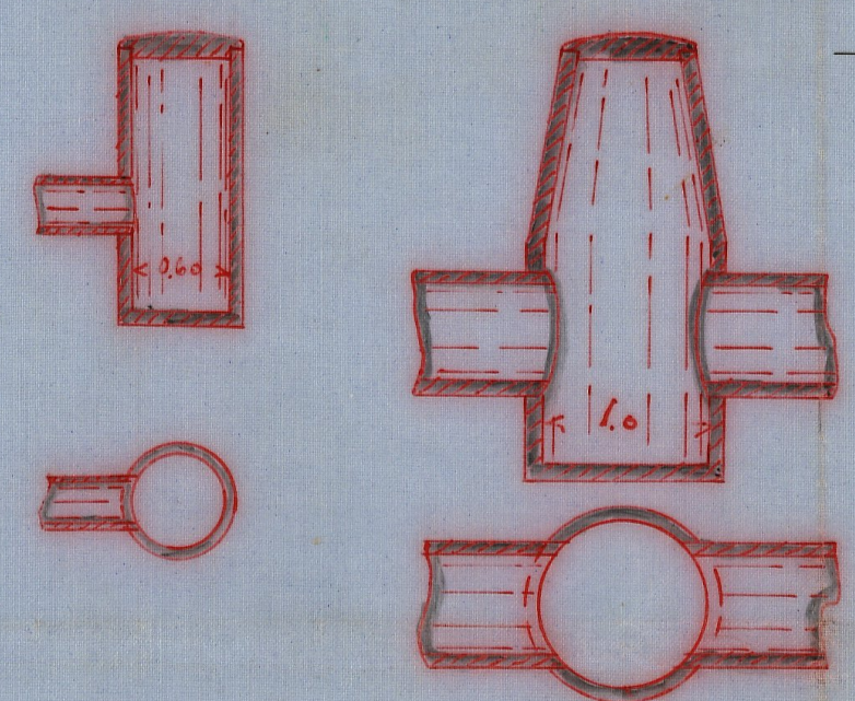
Förslag till brunn. Skala 1:50.
