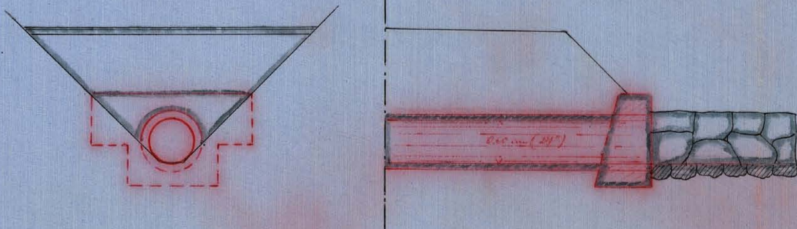
Förslag till ägarevägbro sk. 1:50
