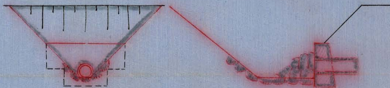
Förslag till ommurning av utloppsror. sk. 1:50
