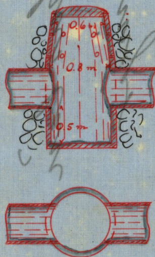
Förslag till 0.8 m. brunn. Skala 1:50.
