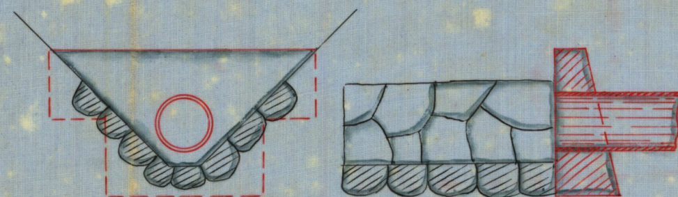
Förslag till omringning. Skala 1:50.
