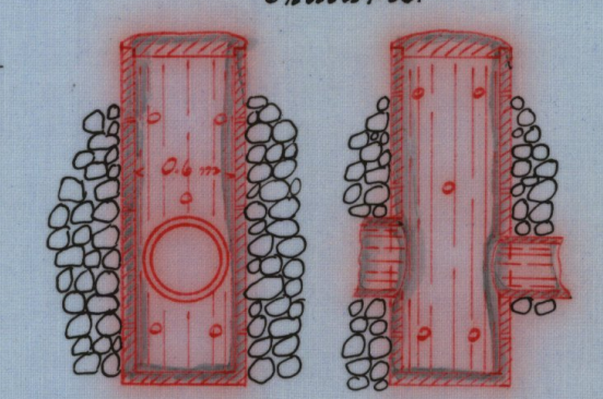
Förslag till brunn. Skala 1:50.
