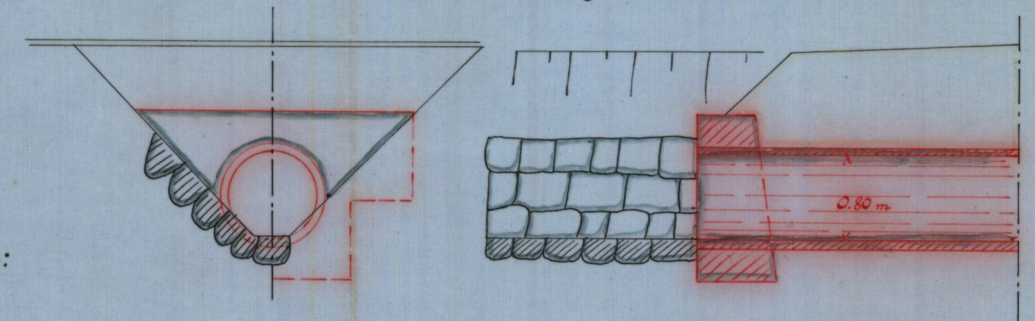
Förslag till älgvägsstrumma vid 16+42. Skala 1:50.
