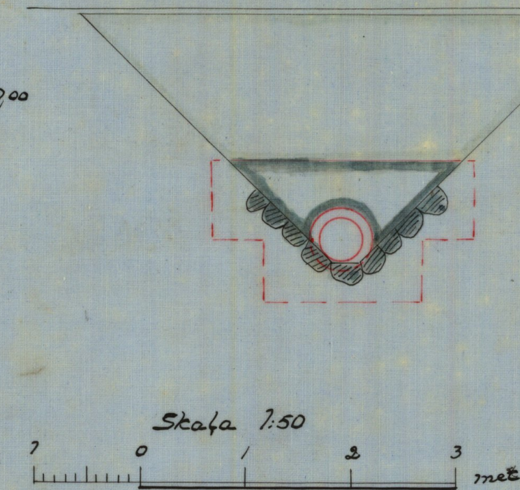
Förslag till brunn. Sk. 1:50
