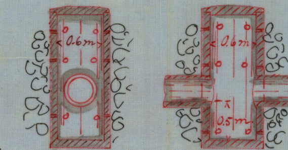
Förslag till brunn. Sk. 1:50
