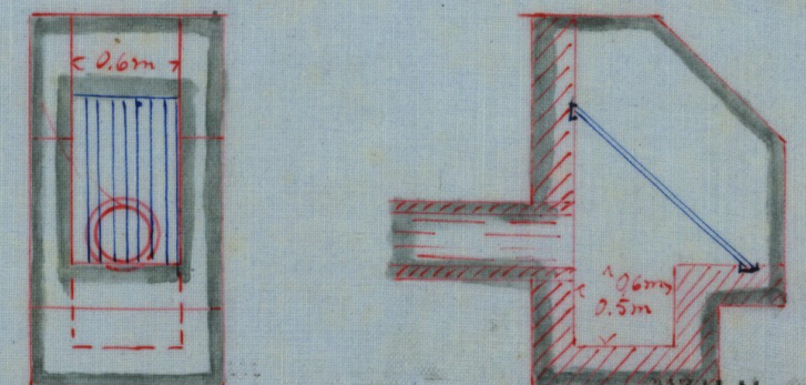
Förslag till intag vid 10+17 Skala 1:50
