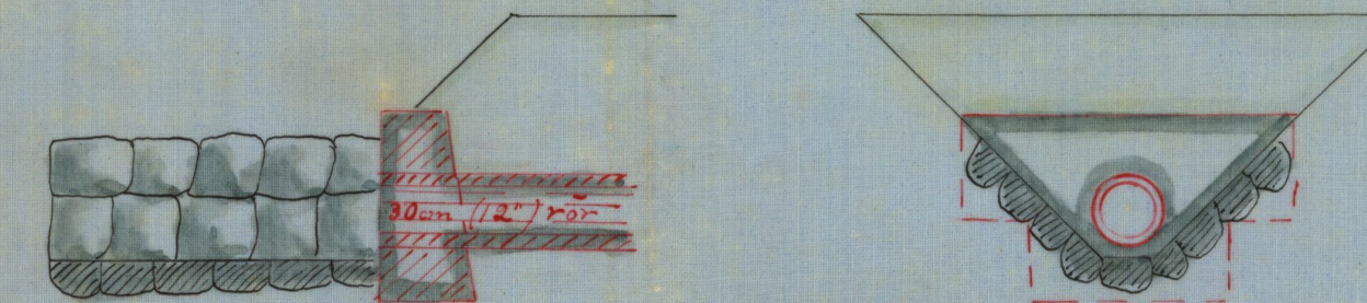
Förslag till kringmurning av utlopp vid 11+6 Sk. 1:50
