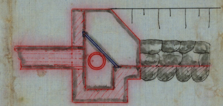
Förslag till inlag Skala 1:50
