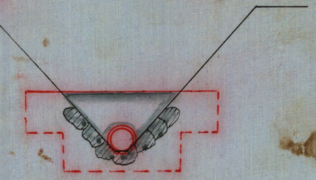
Förslag till ommurning av utlopp Skala 1:50
