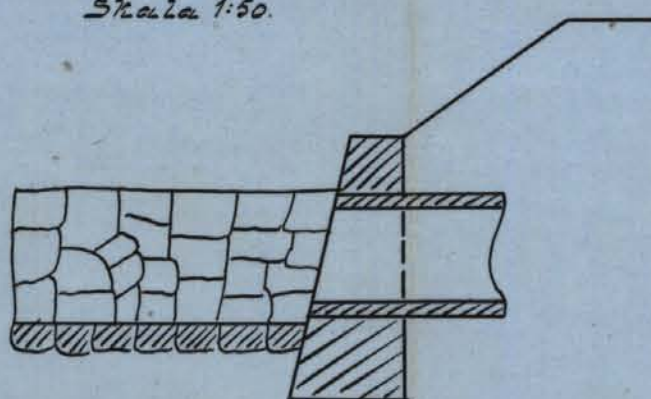
Kringmurning vid H. Skala 1:50.
