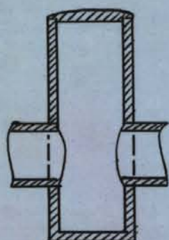
Förslag till brunn. Skala 1:50.
