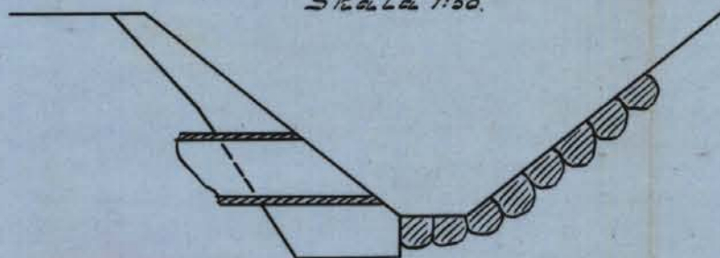
Kringmurning vid F. Skala 1:50.
