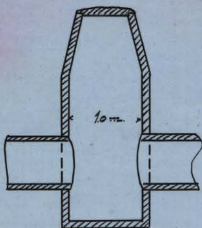
Förslag till brunn. Skala 1:50 1.0 m diam.
