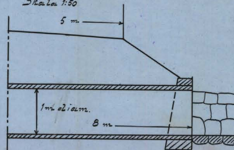
Bro vid 4+92. Skala 1:50.
