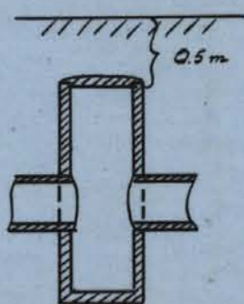
Förslag till brunn. Skala 1:50 1.0 m diam.
