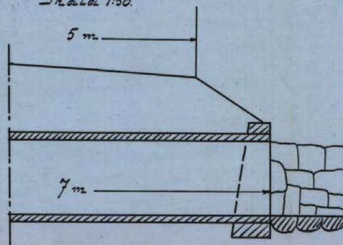
Bro vid 2+65. Skala 1:50.
