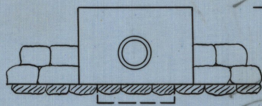
Förslag till kringmurning. Skala 1:50.
