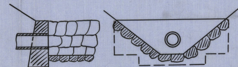
Murning omkärning rörmurning. Skala 1:50.
